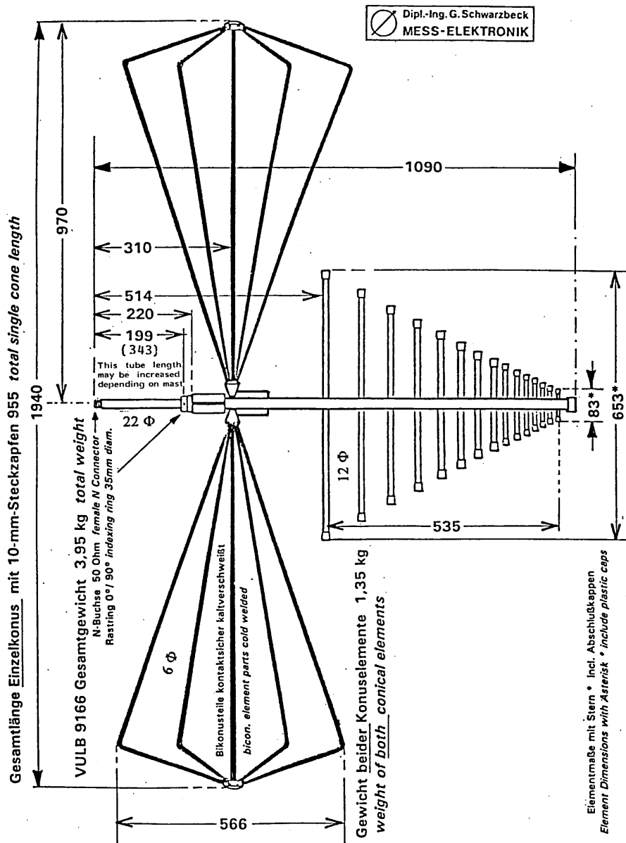
VULB 9166 (9165) Abmessungen und Gewichte LOGBICON Dimensions (mm) and weight (kg)
